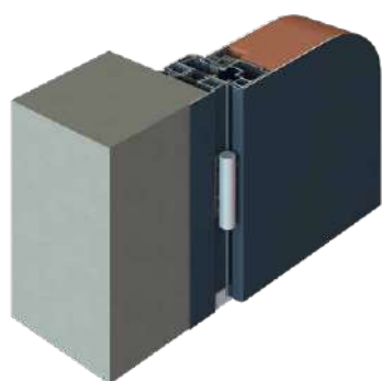
POSE EN BORDS TABLEAU Dormant étroit sans aile + plat de finition
